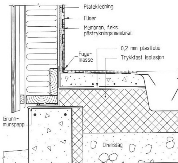
Figur 3.9 Eksempel på våtrumsgolv på grund med ringmur og yttervägg av träregekonstruksjon. Membranen på ytterväggen ersätter ångspärren bakom plattbeklädnaden, (Våtrumsgolv i kjeller og på grunnen 31.206, fig 22 b).
