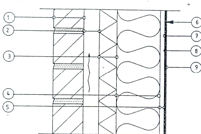
Figur 5.2 Våtrumsyttervägg med träreglar.
