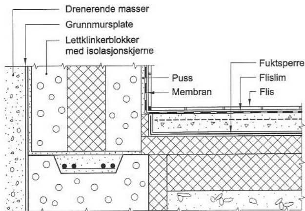
Figur 3.4 Källarvägg av lettklinkerblock med isolerkärna, (Bad i underetasjer 30.055, fig 23 a).
