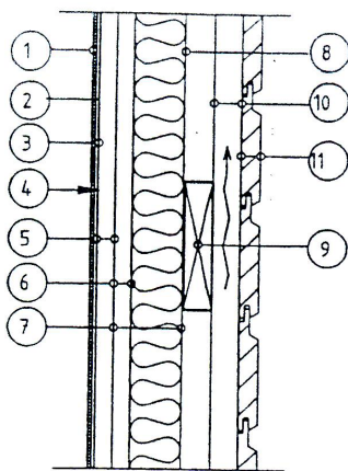
Figur 5.3 Vägg mellan bastu och badrum – gips.
